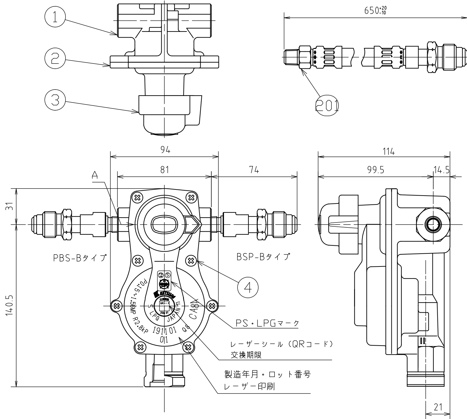
A矢視図
