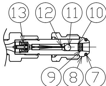
B 詳細
