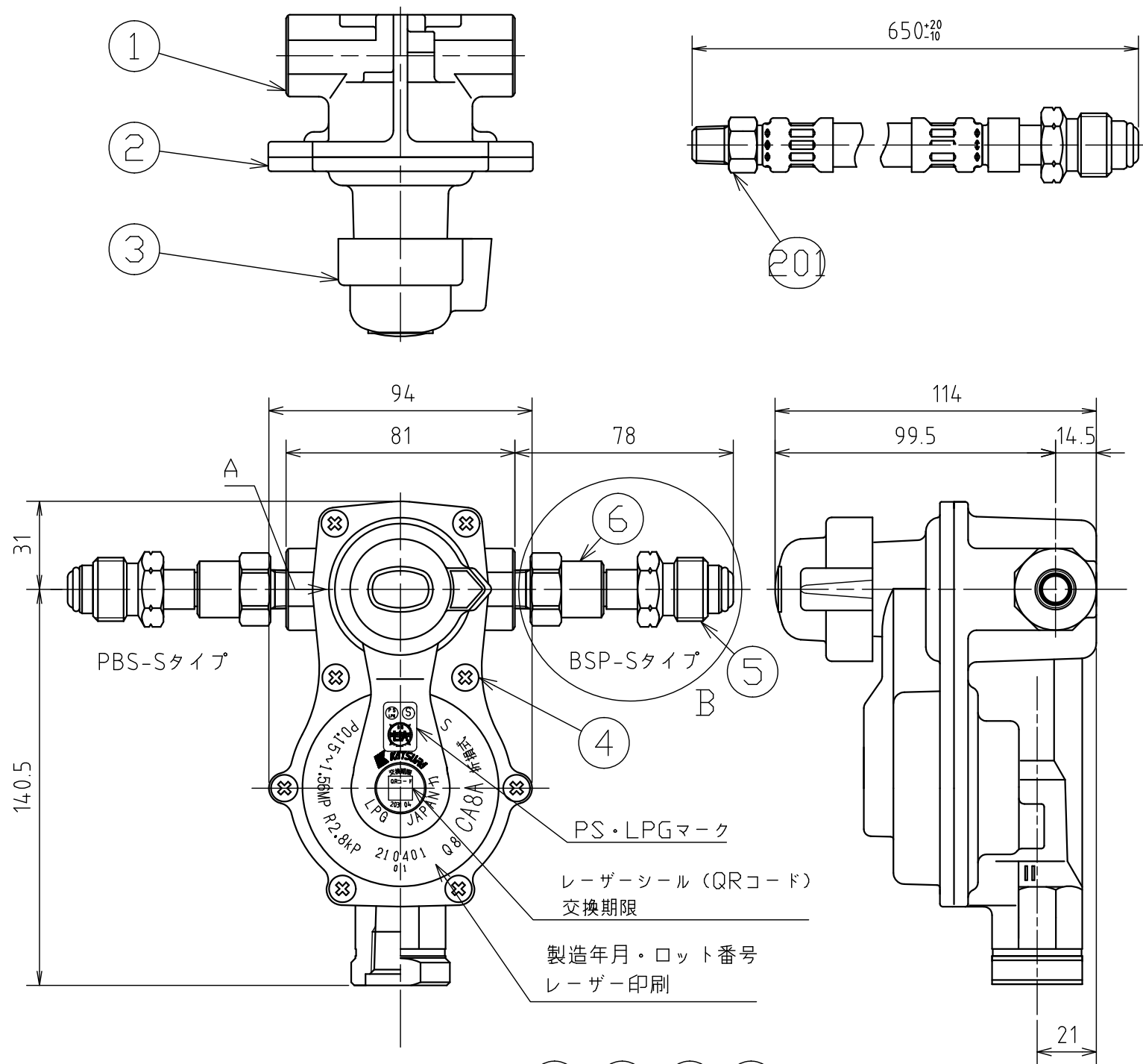
A 矢視図
